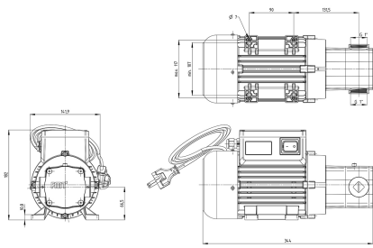
23433 005 Dieselpumpe 100 l/min/26,4USgal - 220 V-1-AC-60 Hz
